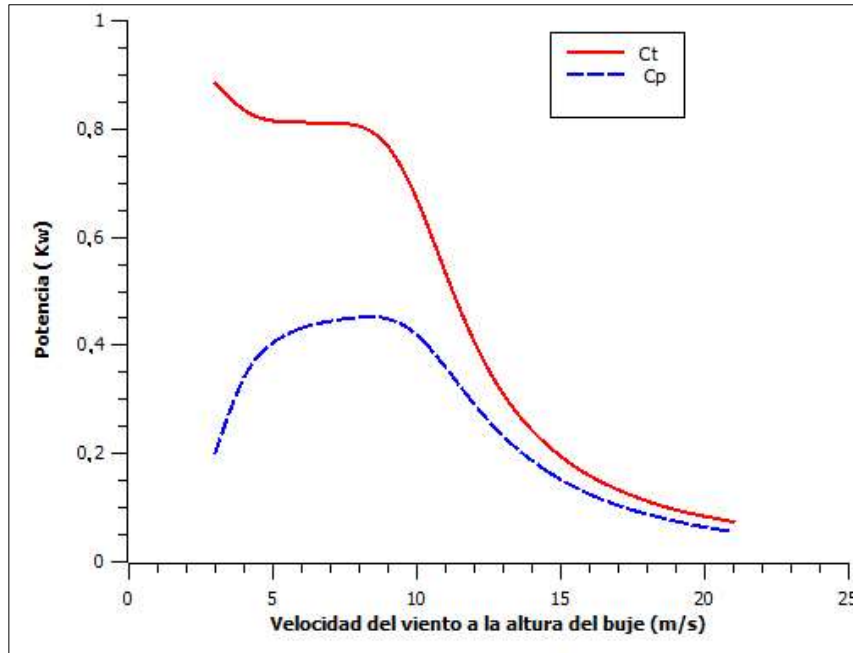
Figura 40. Curvas coeficiente de potencia y coeficiente de empuje modelo Gamesa G90
