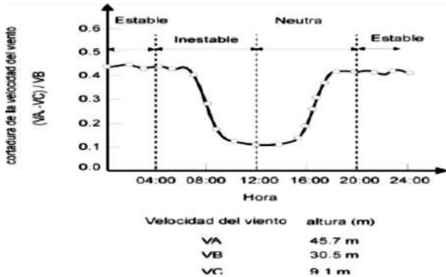
Figura 5. Variación del viento con la altura. Estabilidad atmosférica
