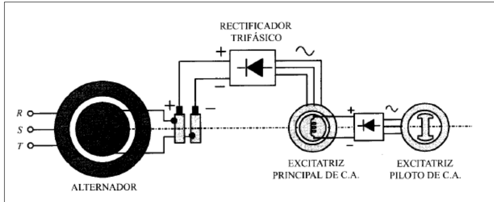
Figura 29. Sistema de excitación electrónico en generadores sincronos
