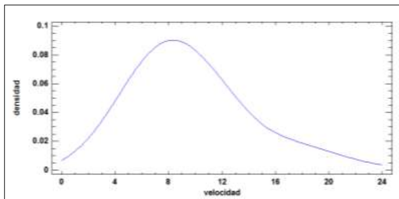
Figura 24. Función de densidad de la velocidad del viento
