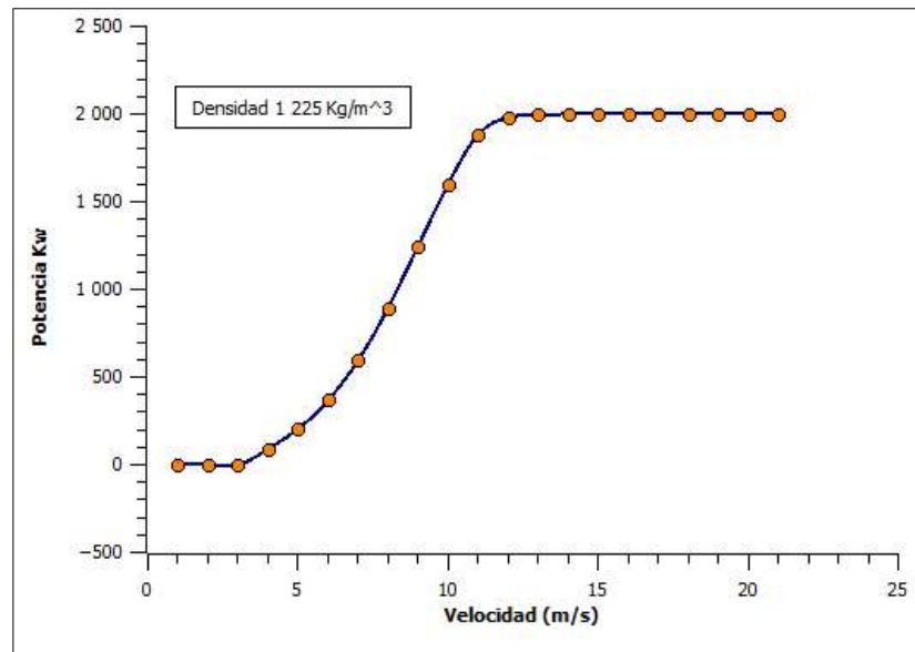
Figura 37. Curva de potencia especifica Vestas Modelo V90-2.0 MW (opción C)
