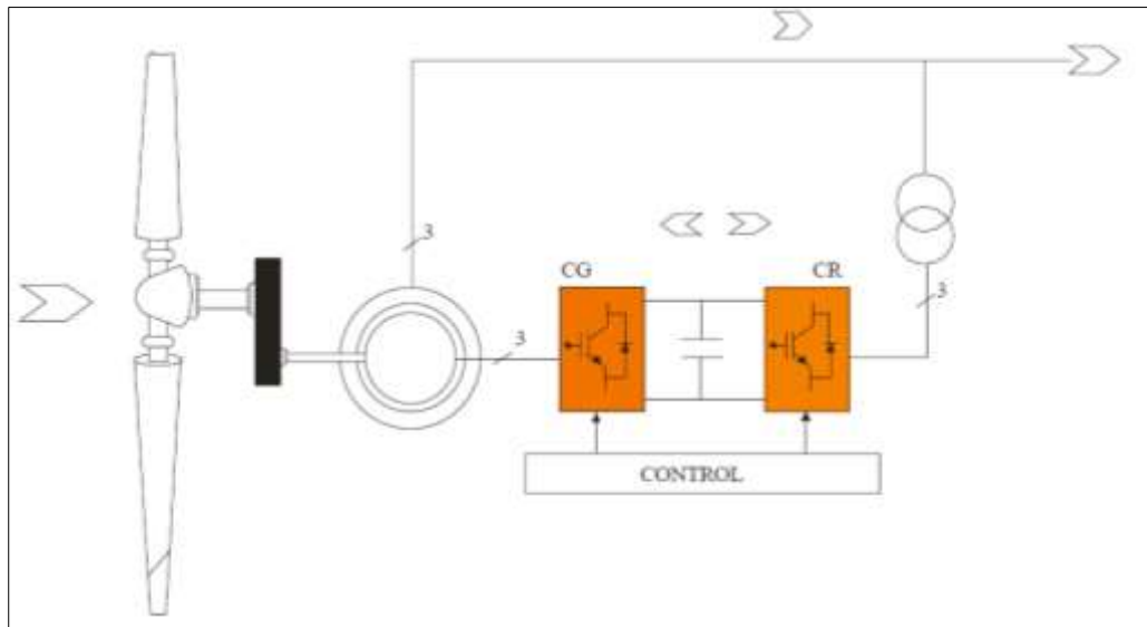
Figura 28. Generador asíncrono de doble alimentación con convertidores electrónicos IGBT
