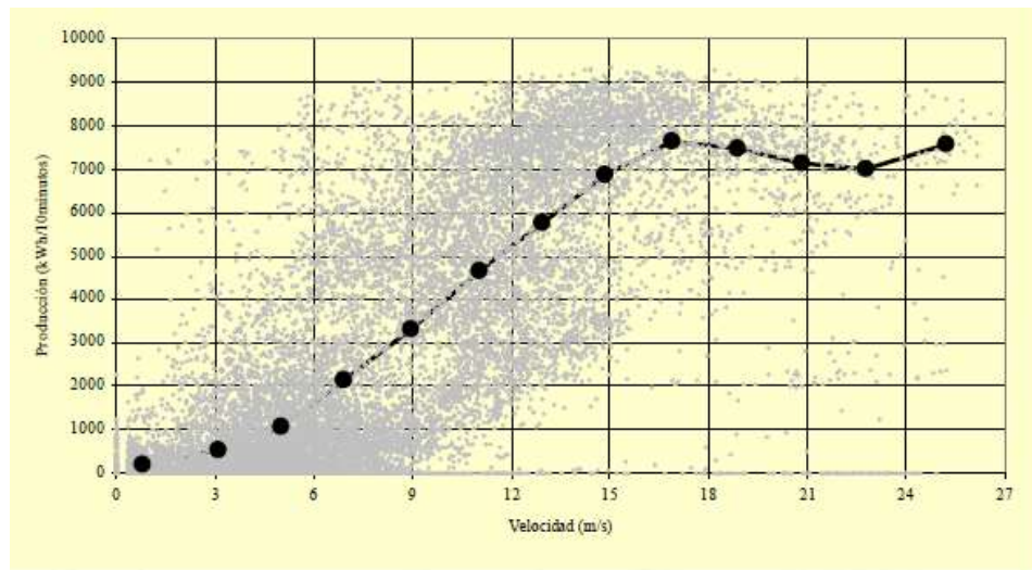
Figura 8. Incertidumbre en mediciones de curvas de potencia
