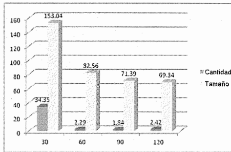
Gráfica 9.3.2.4 Atrás
