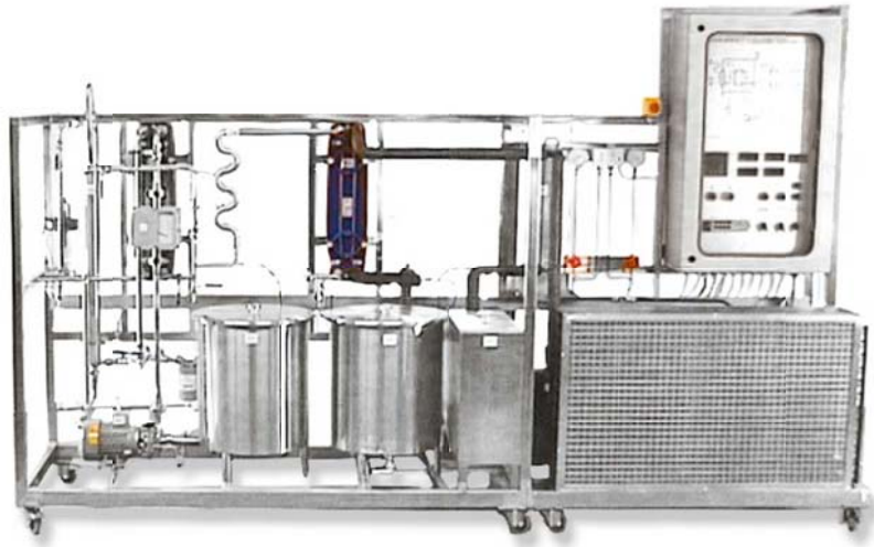
Figura 49. Fotografía pasteurizador
