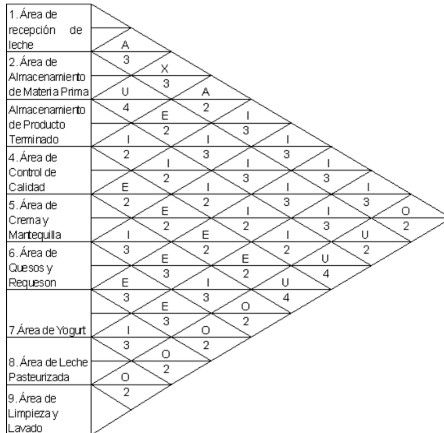
Figura 24. Diagrama de Relación de actividades para las áreas de la planta de elaboración de productos lácteos.
