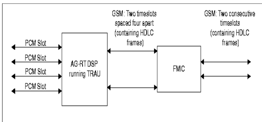
Figura 2. Arquitectura TRAU
