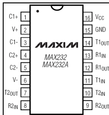
Figura 12. Integrado MAX 232
