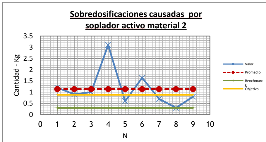
Figura 49. Cantidad de kilogramos sobredosificados en n muestras al estar activado el soplador neumático en el material 2
