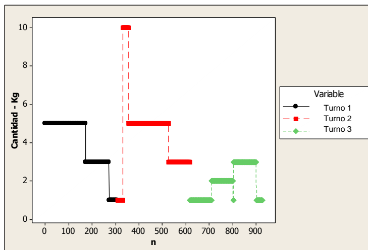
Figura 19. Gráfico del cambio de parámetro de tolerancia por turno del material 4
