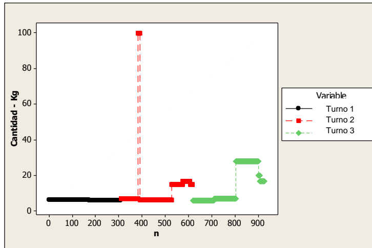
Figura 18. Gráfico del cambio de parámetro de error de caída por turno del material 3
