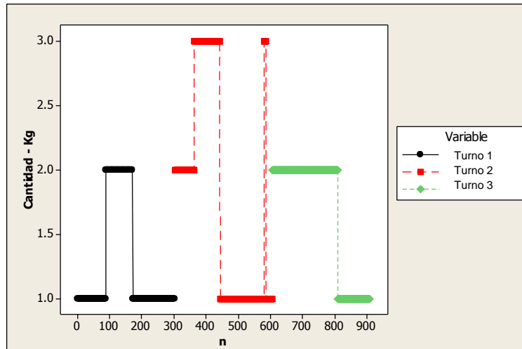
Figura 10. Gráfico del cambio de parámetro de tolerancia por turno del material 1
