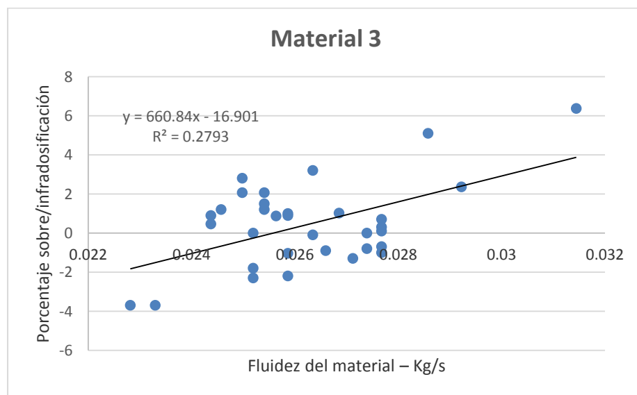
Figura 45. Gráfico de porcentaje sobre/infradosificación frente a fluidez del material 3
