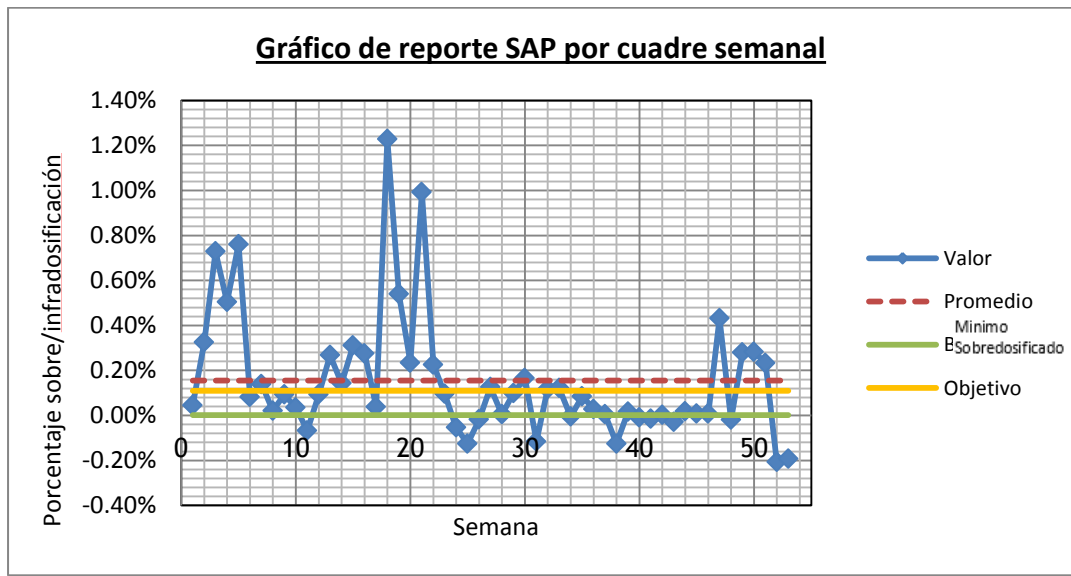
Figura 5. Gráfico de comportamiento del material número 2
