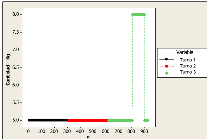
Figura 16. Gráfico del cambio de parámetro de tolerancia por turno del material 3
