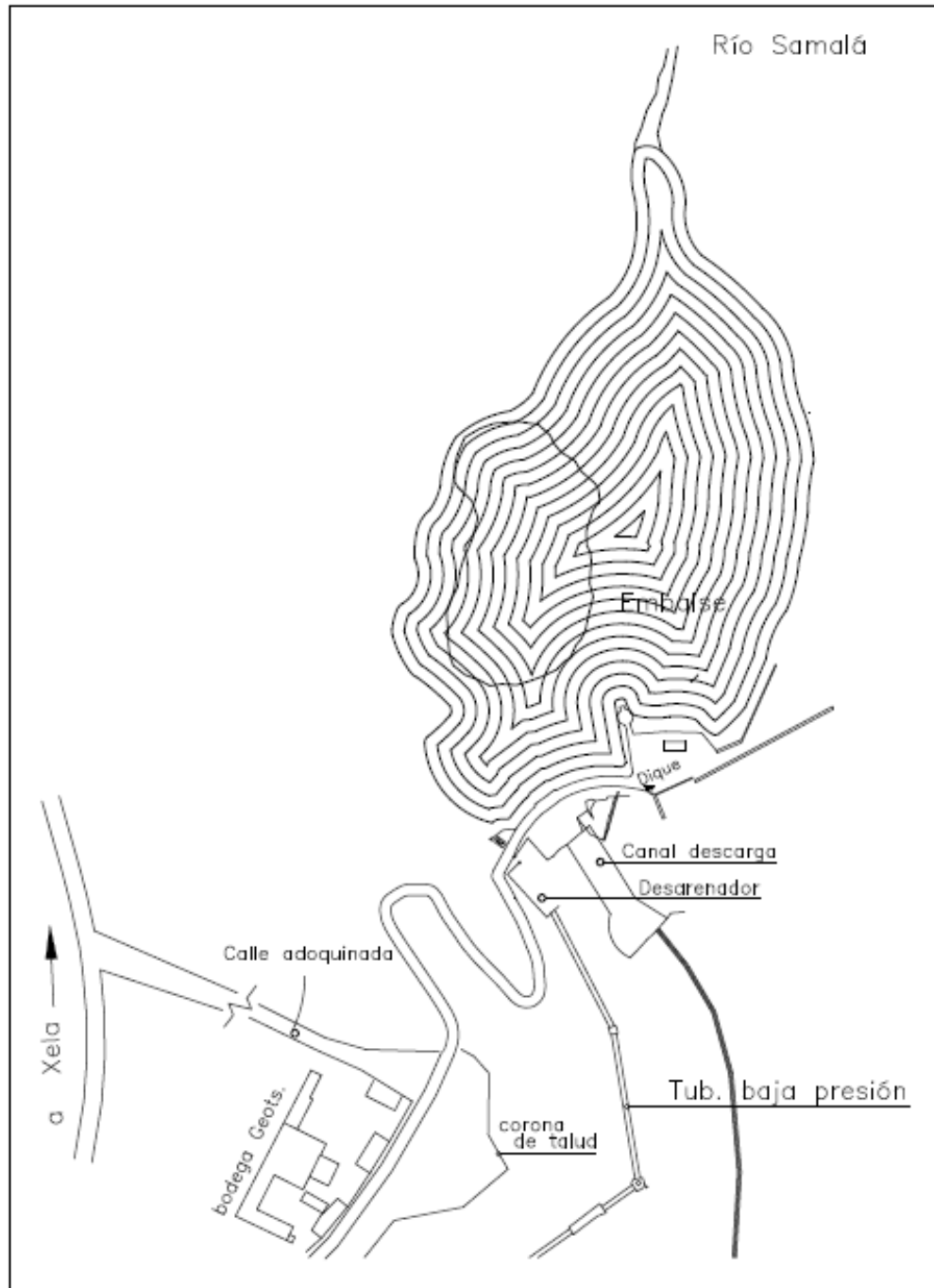
Figura 3. Ubicación y vías de acceso proyecto hidroeléctrico Santa María
