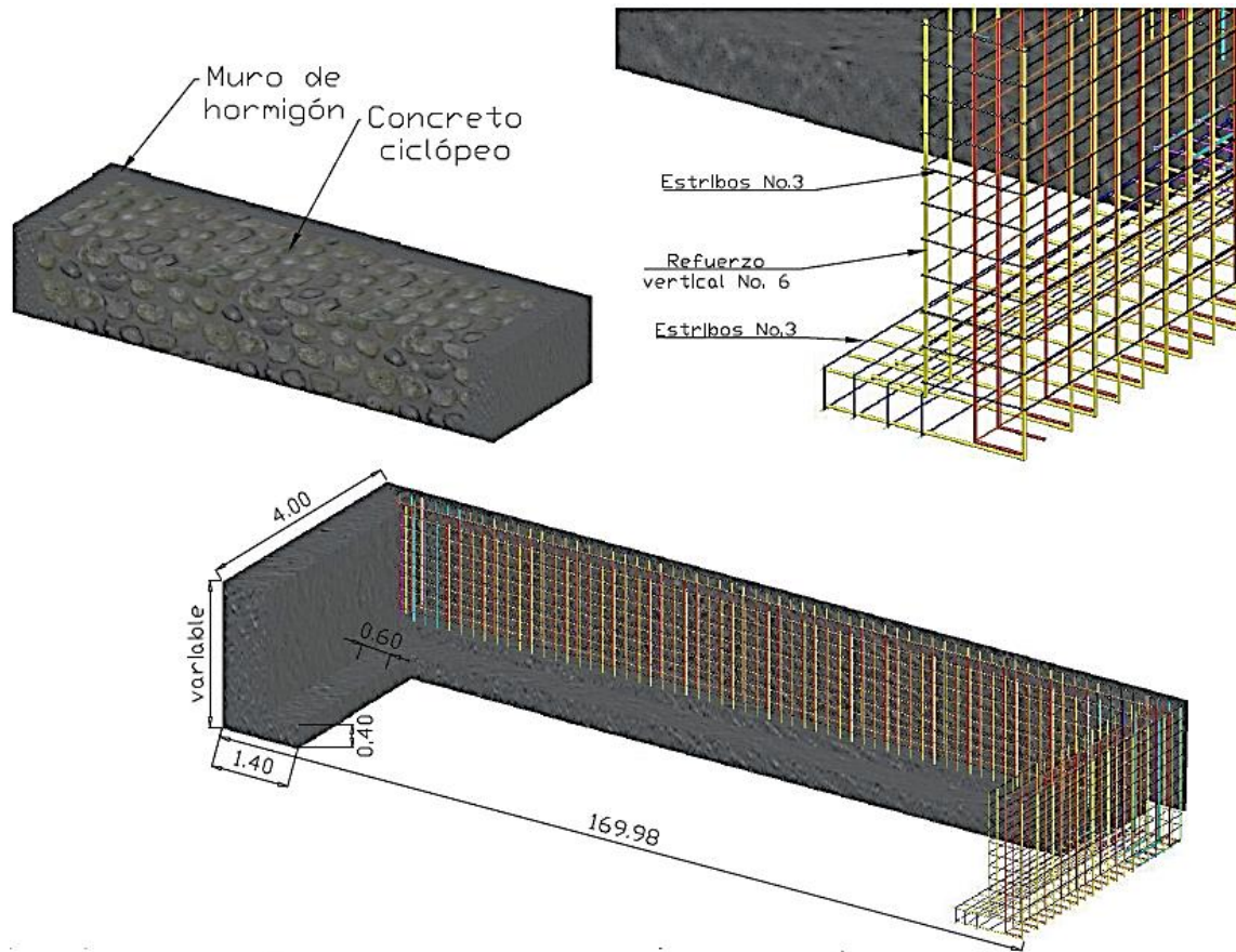
Figura 39. Armado de muro de anclaje
