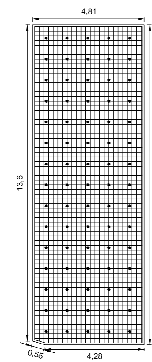
Losa No. 8 Área = 66.05 m 2
