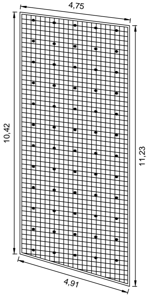
Losa No. 4 Área = 50.99 m 2
