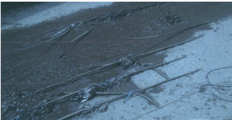
Figura 12. Refuerzo expuesto en losa del canal de desfogue
