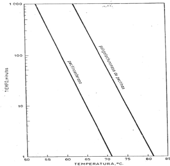
Figura 9. Temperatura de inactivación para la poligalacturonasa y la pectinesterasa de un preparado enzimático comercial
