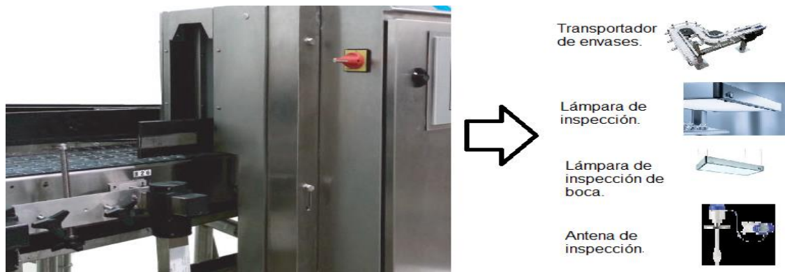
Figura 56. Modelo de mantenimiento del inspector electrónico
