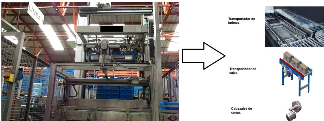
Figura 51. Modelo de mantenimiento preventivo de la despaletizadora
