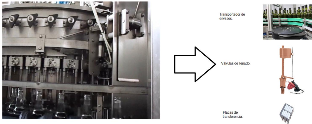
Figura 57. Modelo de mantenimiento preventivo de la llenadora
