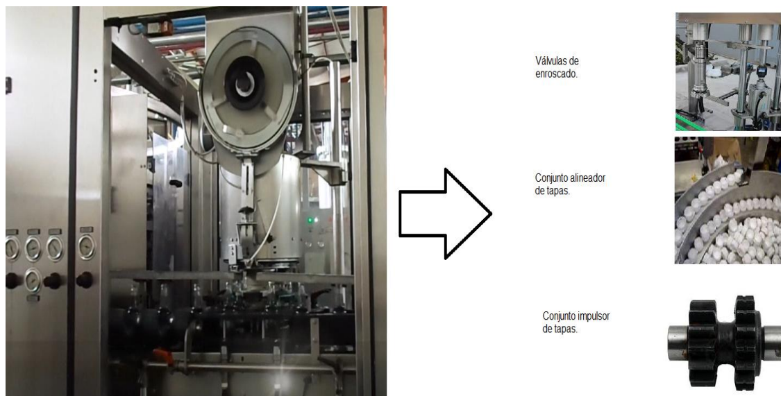
Figura 58. Modelo de mantenimiento preventivo de la taponadora
