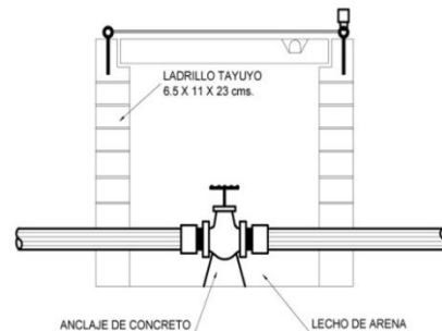
Sección.
