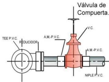
Elevación.
