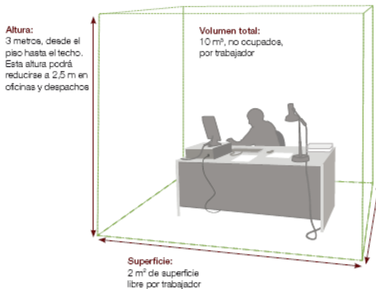
Ilustración No. 03 Dimensiones mínimas de locales de trabajo Fuente: Folleto de Diseño del puesto de trabajo en oficinas en las administraciones públicas
