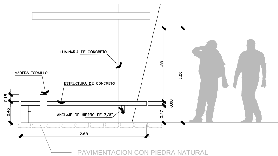
ELEVACION FRONTAL BANCA TIPICA
