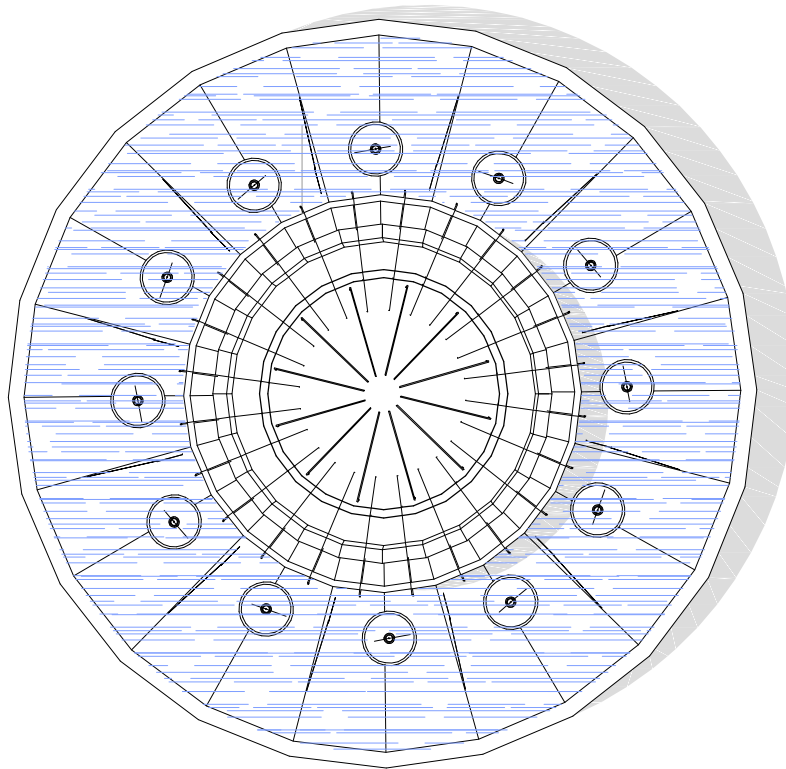
PLANTA ARQUITECTONICA FUENTE 02
