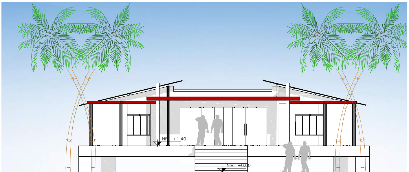
ELEVACION FRONTAL BUNGALOW
