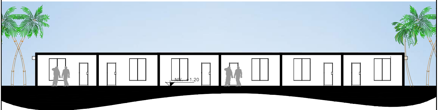
SECCION C - C' ÁREA DE HABITACIONES
