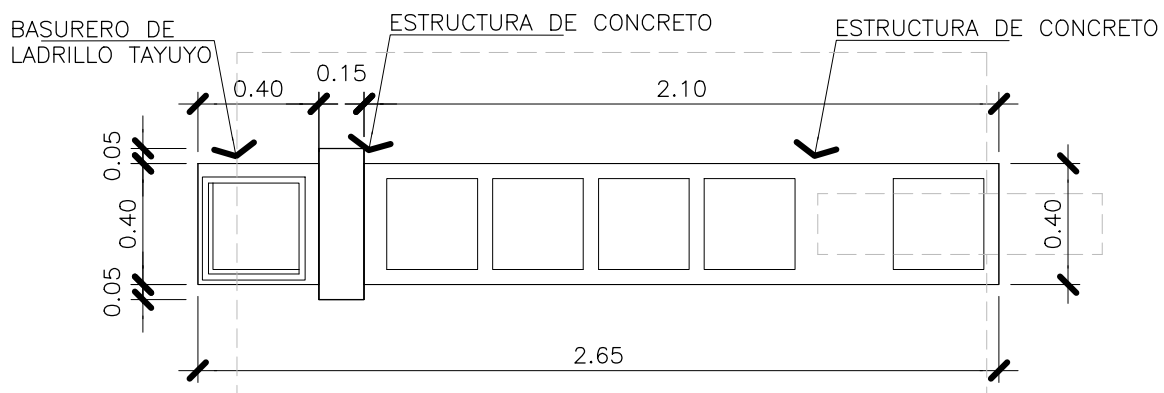
PLANTA ARQUITECTONICA BANCA TIPICA
