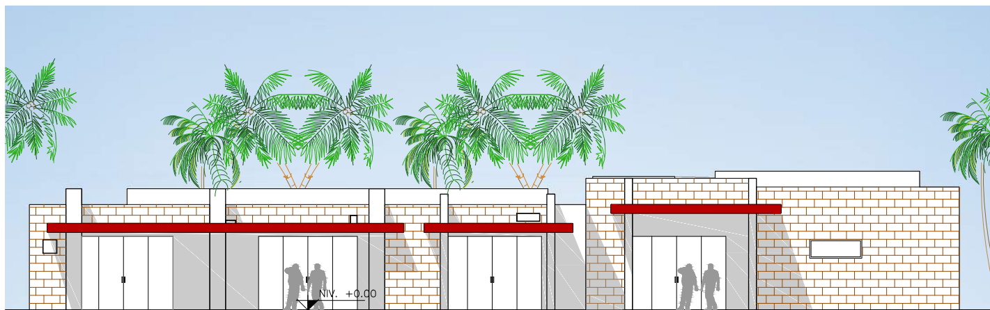
ELEVACION ESTE ÁREA DE EXPOSICIONES ESC: 1/200
