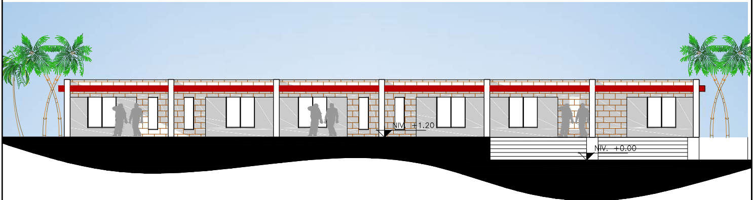
ELEVACION NOR ESTE ÁREA DE HABITACIONES
