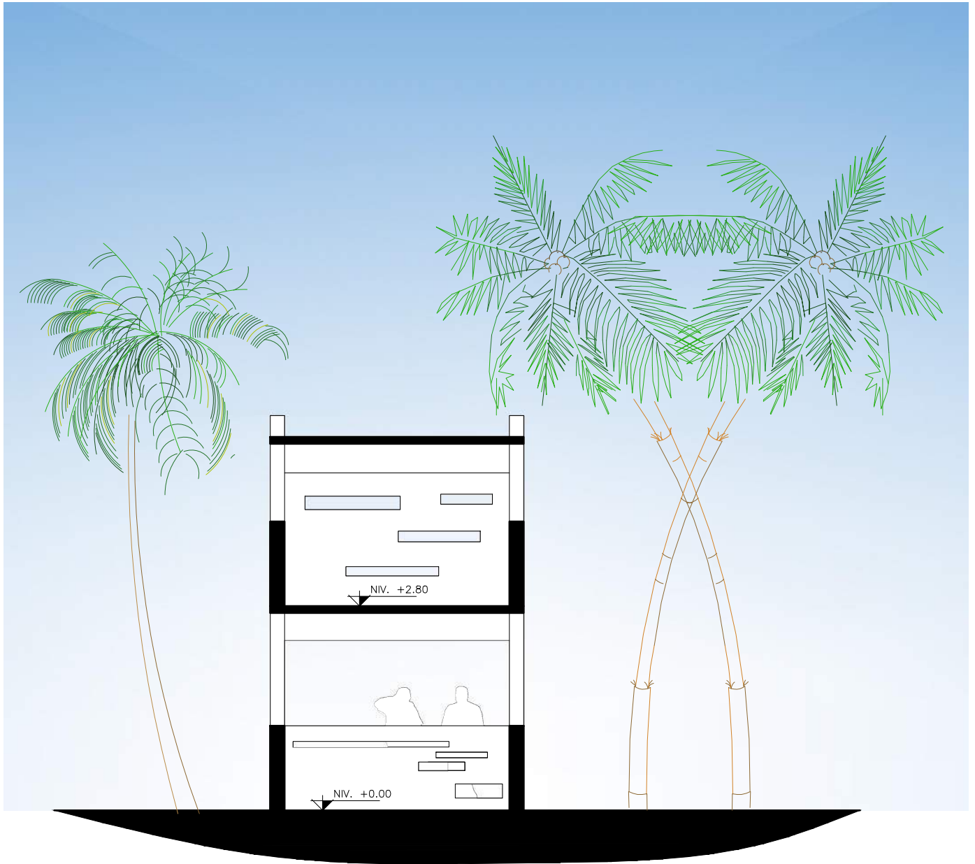
SECCION A - A' MIRADORES (BAMBÚ) ESC. 1/75
