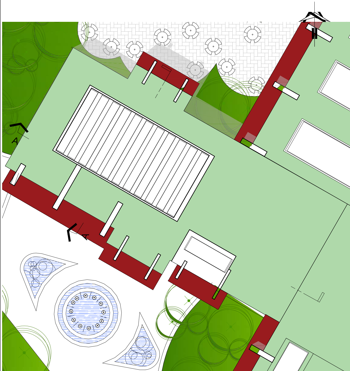
PLANTA DE TECHOS ÁREA DE EXPOSICIONES
