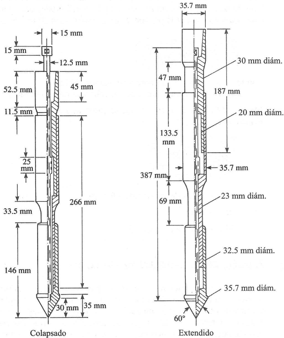
Figura 22. Penetrómetro de cono de fricción mecánica según la ASTM, 1997
