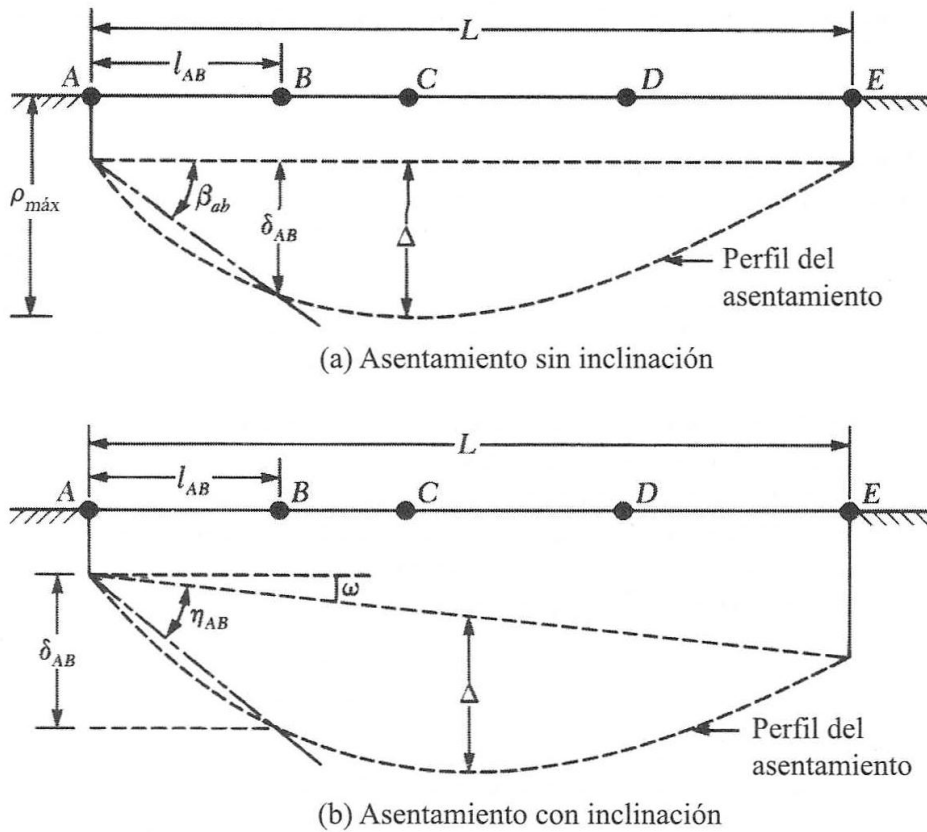
Figura 70. Parámetros para la definición tolerable (según Whals, 1981; redibujado)
