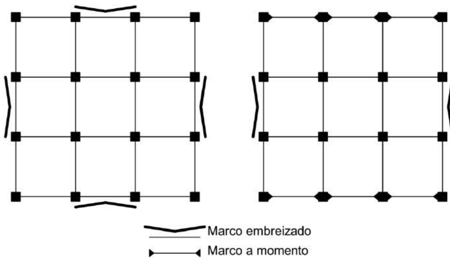
Figura 2. Rigidez lateral en ejes externos para marcos de acero
