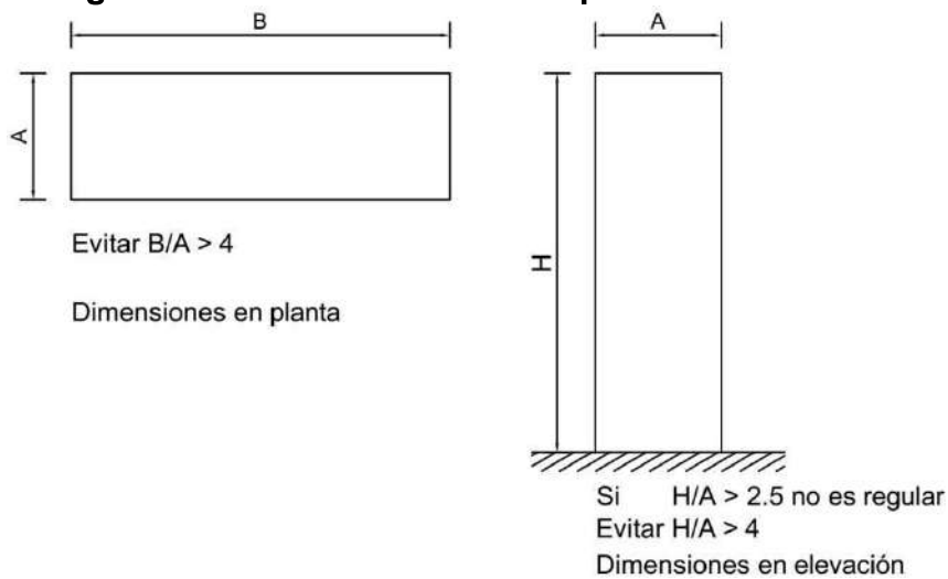
Figura 7. Límites recomendados para los lados en planta y altura en elevación para un edificio, de acuerdo a Normas Técnicas de Diseño por Sismo del Reglamento de Construcciones para el Distrito Federal (NTDS)
