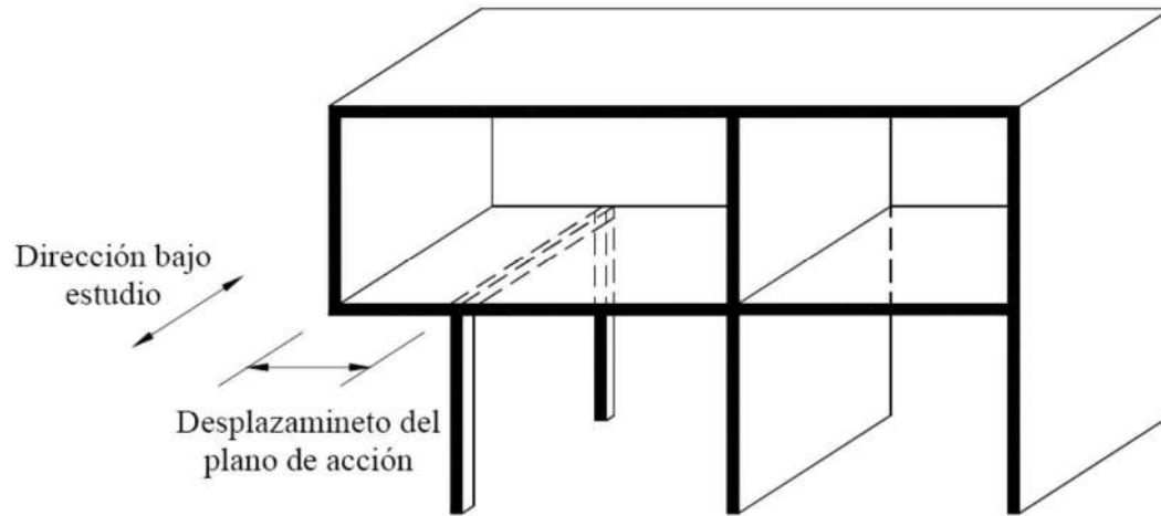
Figura 12. Irregularidad por desviación fuera del plano
