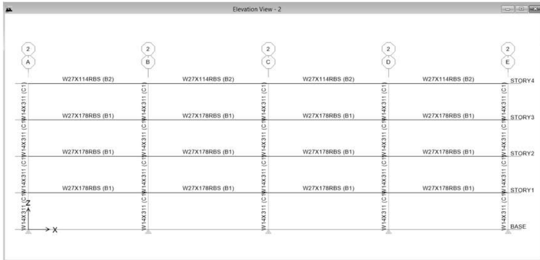
Eje 2/A-E, vigas asignadas como RBS
