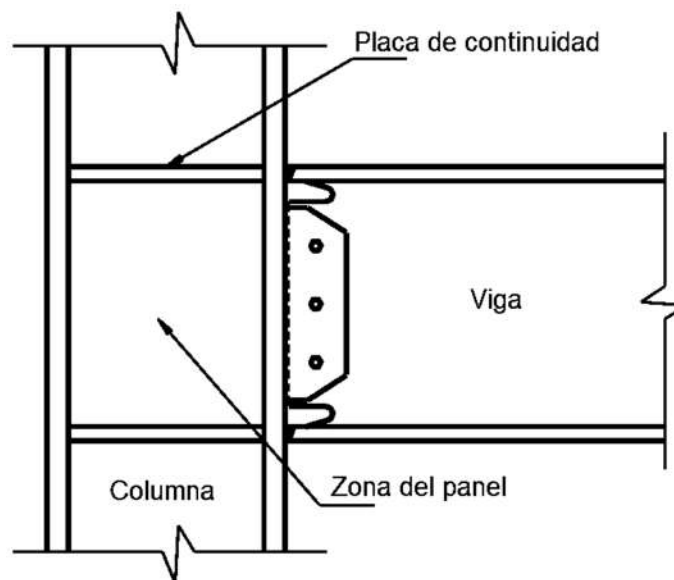
Figura 27. Ubicación de placas de continuidad
