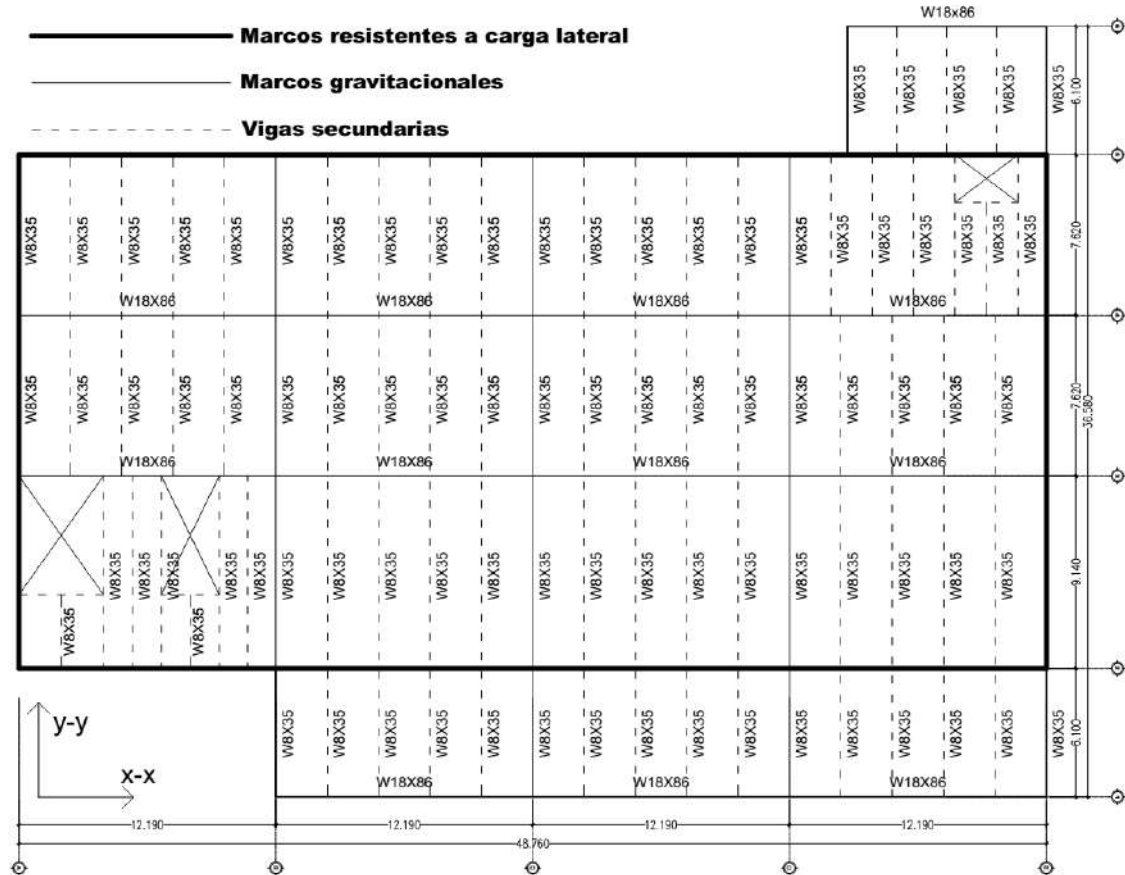
Planta de distribución de vigas nivel 4, de acuerdo con el diseño realizado en los pasos 2.6.1 al 2.6.9 (vigas principales) y 2.7.1 y 2.7.10 (vigas secundarias)
