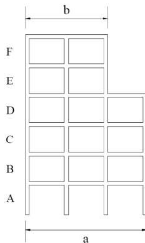
Figura 16. Irregularidad geométrica vertical
