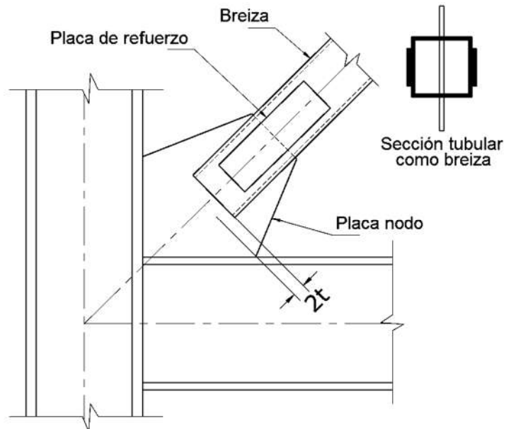
Figura 34. Detalle de conexión con breiza de sección tubular, reforzada con placas, recomendado por AISC 341-10
