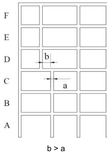
Figura 17. Irregularidad por discontinuidad en el plano de elementos verticales resistentes a fuerzas laterales
