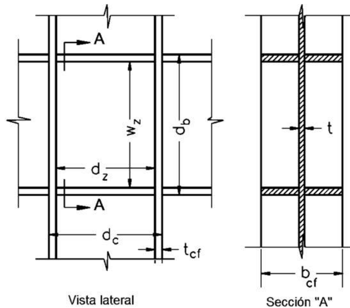
Figura 29. Zona del panel conexión viga – columna
