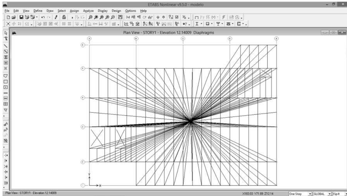
Planta del modelo con el diafragma rígido asignado
