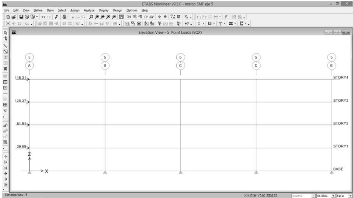
Marco del eje 5 (SMF) modelado en ETABS v9.5
