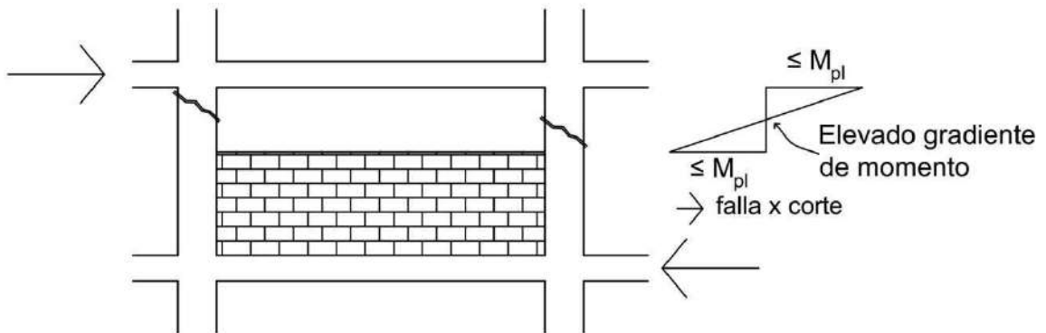
Figura 20. Efectos de columna corta, por ubicación de muros de mampostería de baja altura entre marcos
