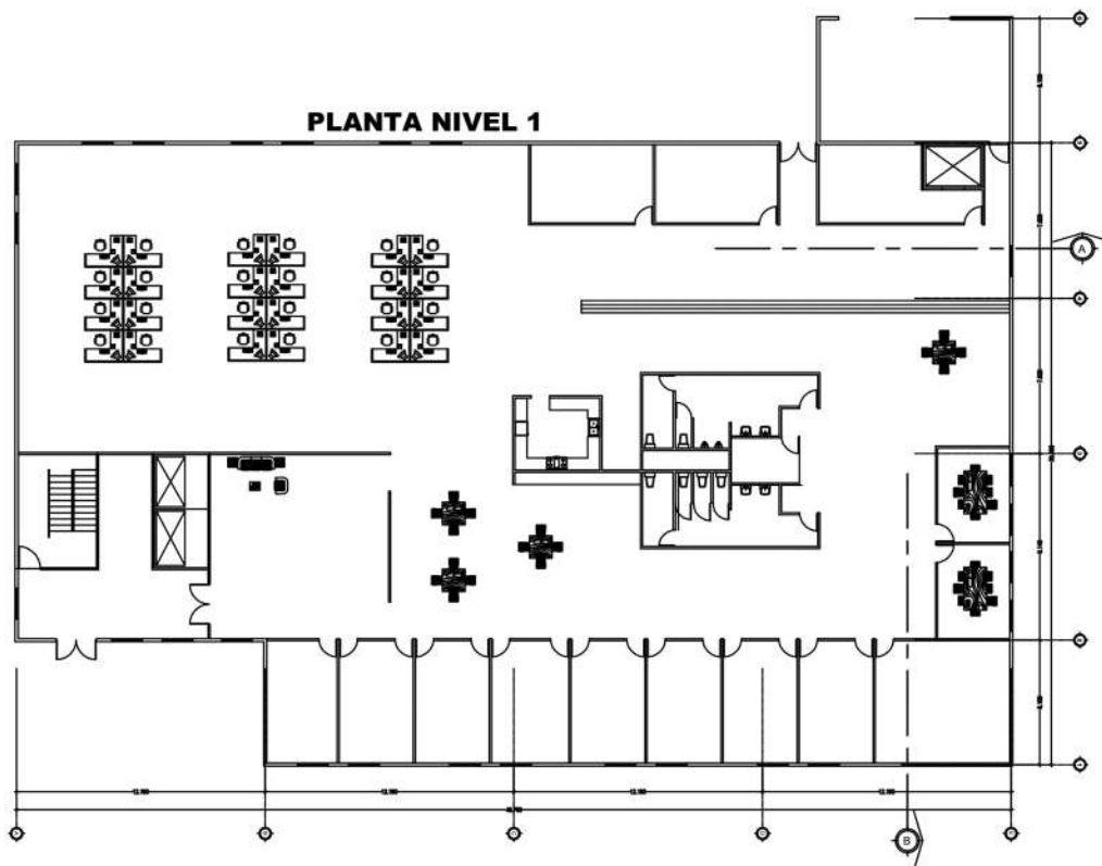
Planta arquitectónica No. 1
