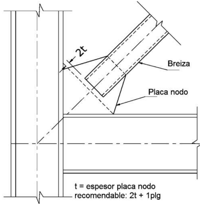
Figura 33. Detalle de conexión recomendado por AISC 341-10
