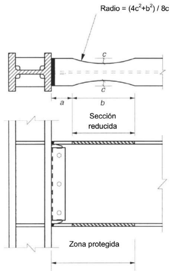
Figura 30. Conexión con viga de sección reducida, RBS
