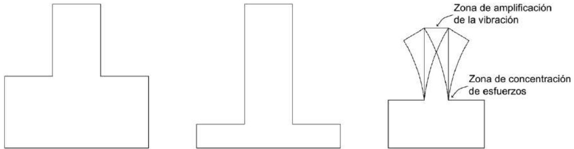
Figura 6. Reducciones no recomendables en pisos superiores de edificios
