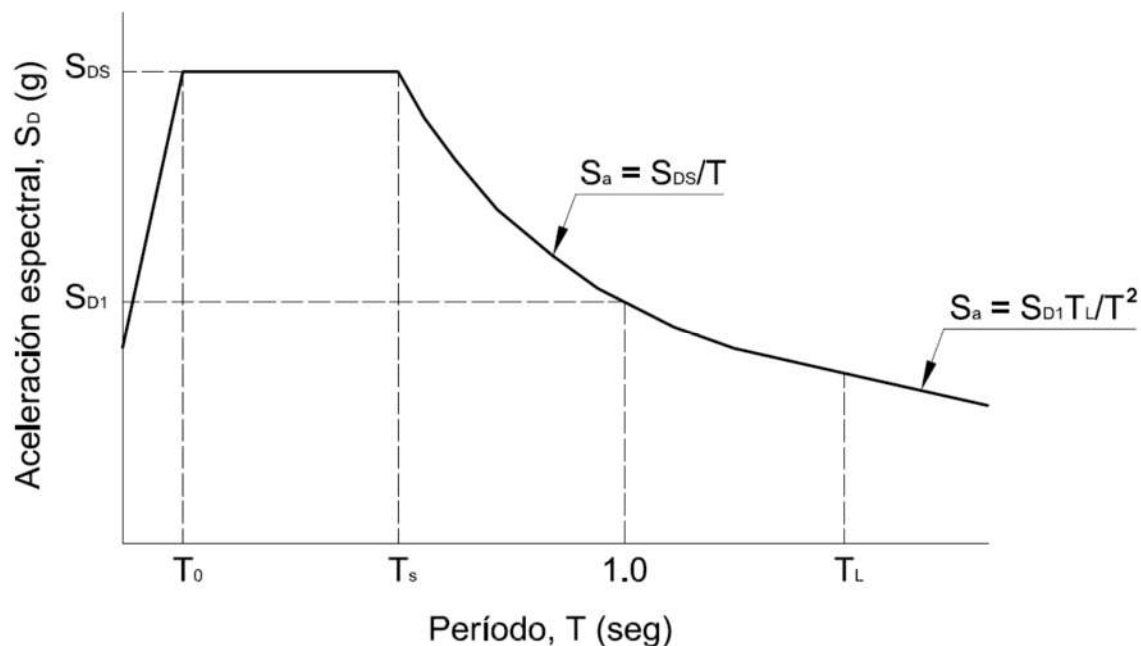
Figura 25. Espectro de diseño
