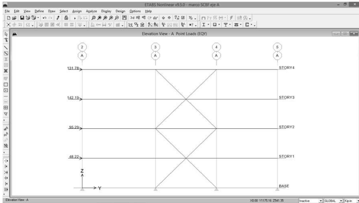
Marco del eje A (SCBF) modelado en ETABS v9.5
