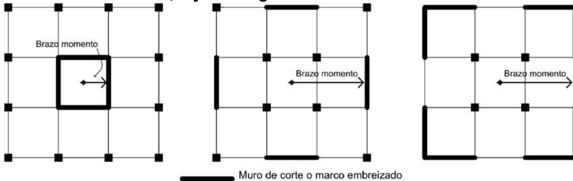
Figura 3. Ubicación de muros de cortante para resistir efectos de volteo y torsión, b y c configuraciones recomendadas
