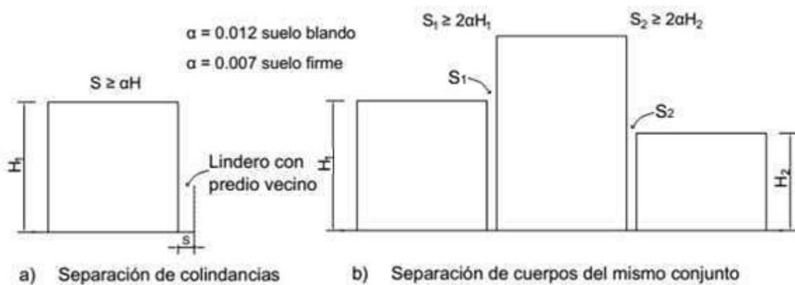
Figura 22. Separación recomendable entre edificios, de acuerdo a Normas Técnicas de Diseño por Sismo del Reglamento de Construcciones para el Distrito Federal (NTDS)
