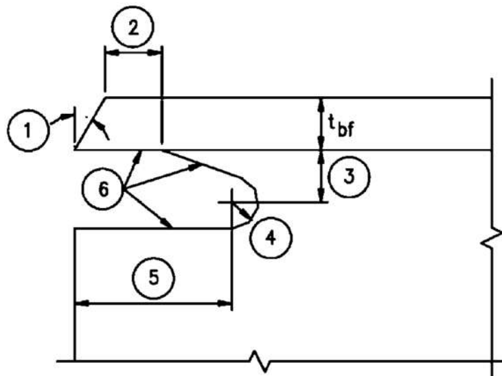
Figura 28. Orificio de acceso para soldadura, FEMA, 2000a
