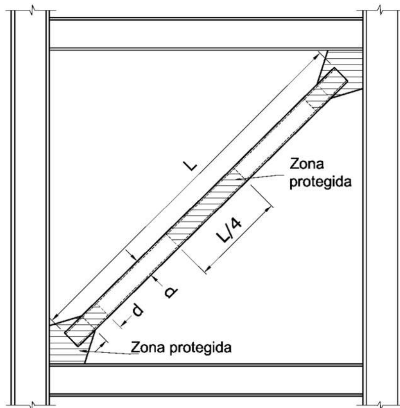
Figura 31. Zonas protegidas en una breiza y sus conexiones
