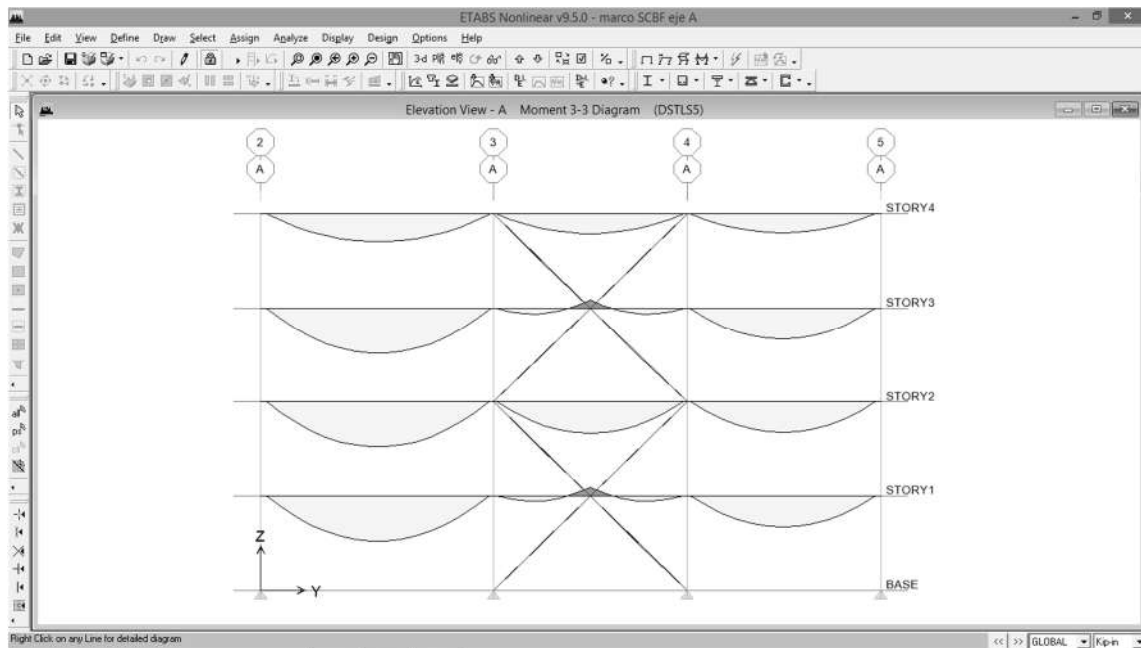
Diagrama de momentos (marco del eje A SCBF)
