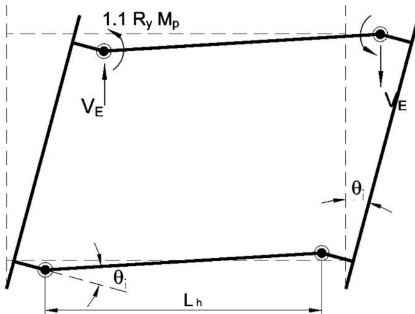
Figura 26. Mecanismo de deformación plástica en articulaciones de vigas
