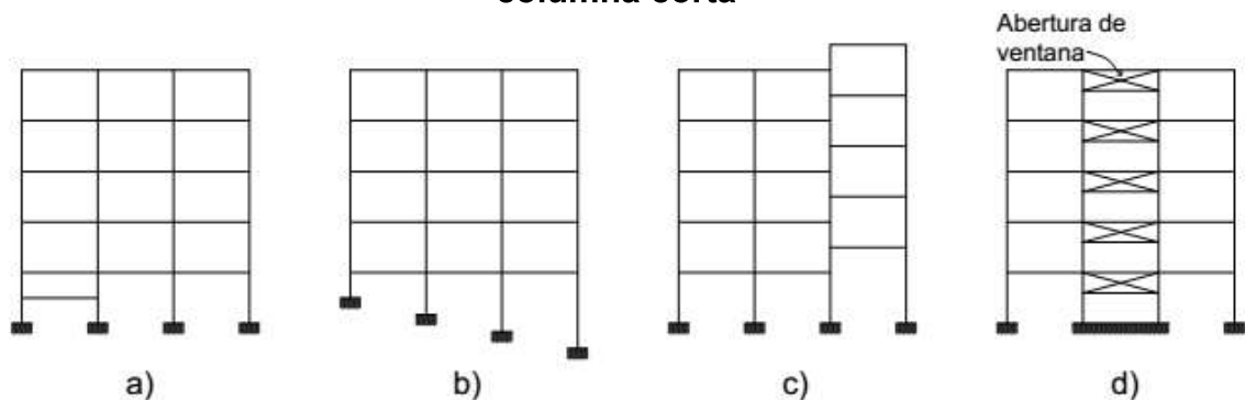
Figura 21. Configuraciones en elevación donde se generan efectos de columna corta
