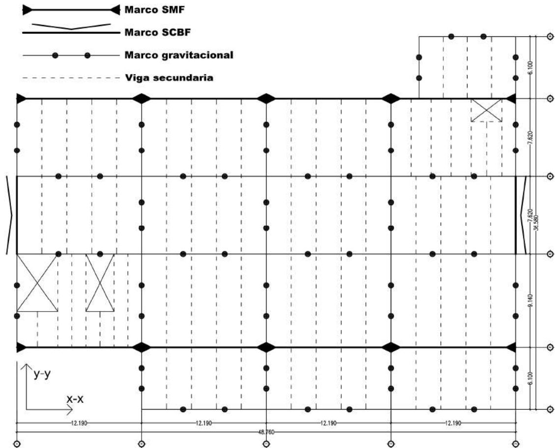
Planta de distribución de marcos para los 4 niveles y ubicación de los sistemas estructurales determinados conforme a los pasos 3.3 y 3.4.
