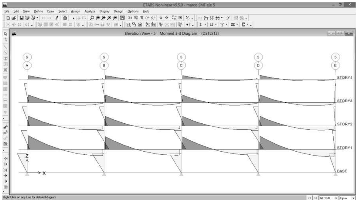
Diagrama de momentos (marco del eje 5 SMF)
