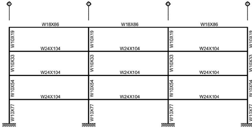
EJE 1 / B-E
