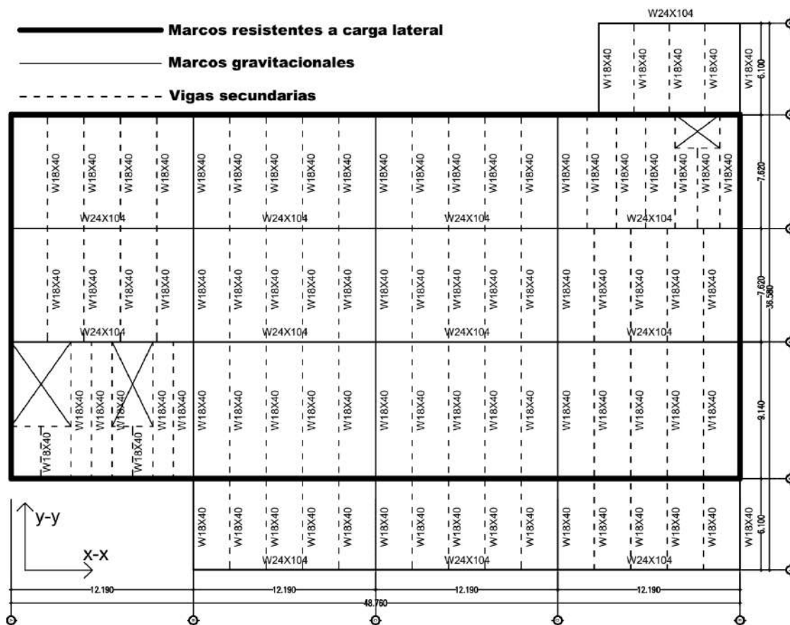
Planta de distribución de vigas nivel 1, 2 y 3, de acuerdo con el diseño realizado en los pasos 2.6.1 al 2.6.9 (vigas principales) y 2.7.1 y 2.7.10 (vigas secundarias)
