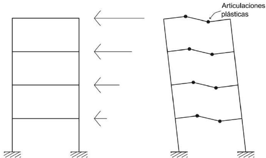
Figura 8. Continuidad de la estructura, ubicación de articulaciones plásticas en la viga para lograr el efecto columna fuerte-viga débil
