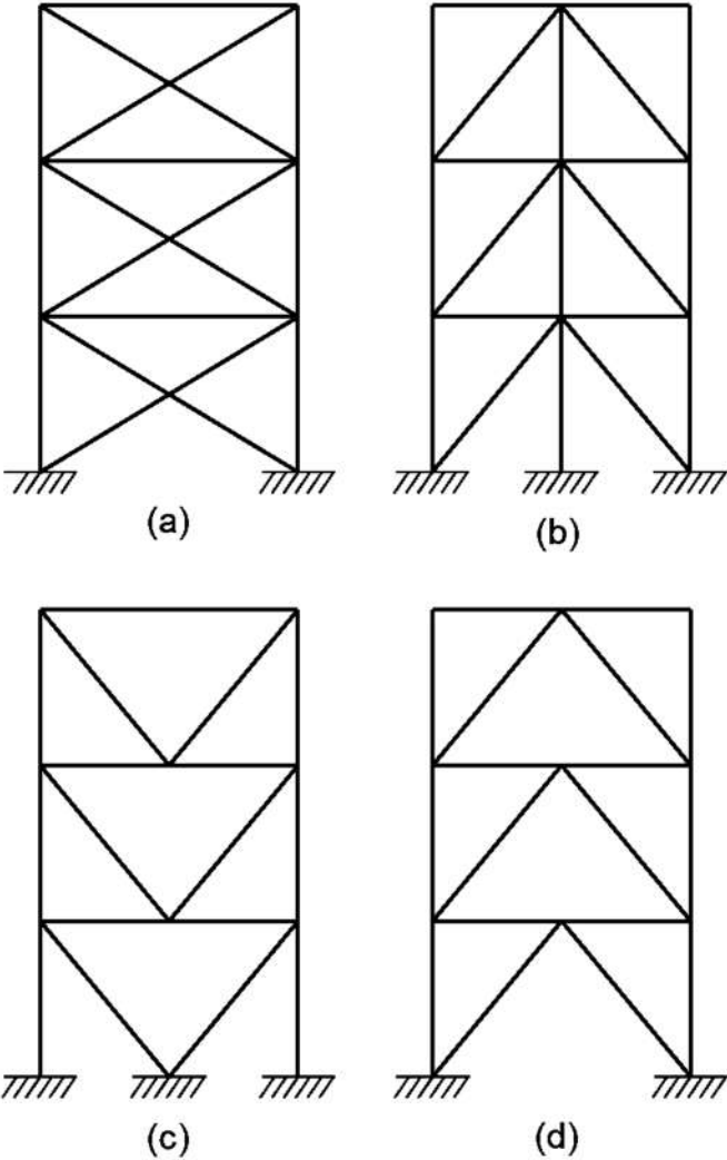
(a) en X, (b) diagonales, (c) en V, (d) en V invertida o Chevron
