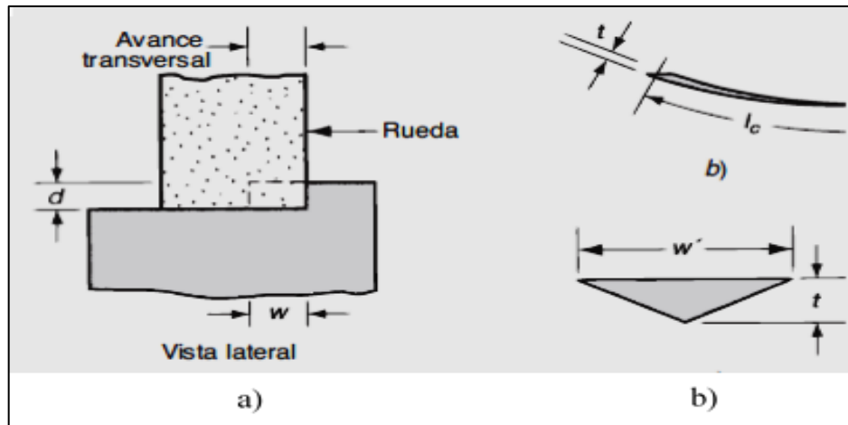
Figura 56. Forma longitudinal y sección transversal de una viruta simple
