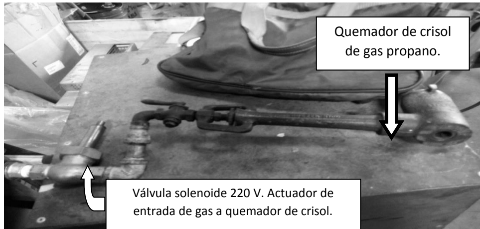
Figura 71. Quemador de crisol de gas propano
