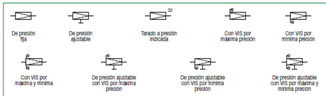
Figura 75. Nomenclatura utilizada en instalaciones de GLP o gas propano
