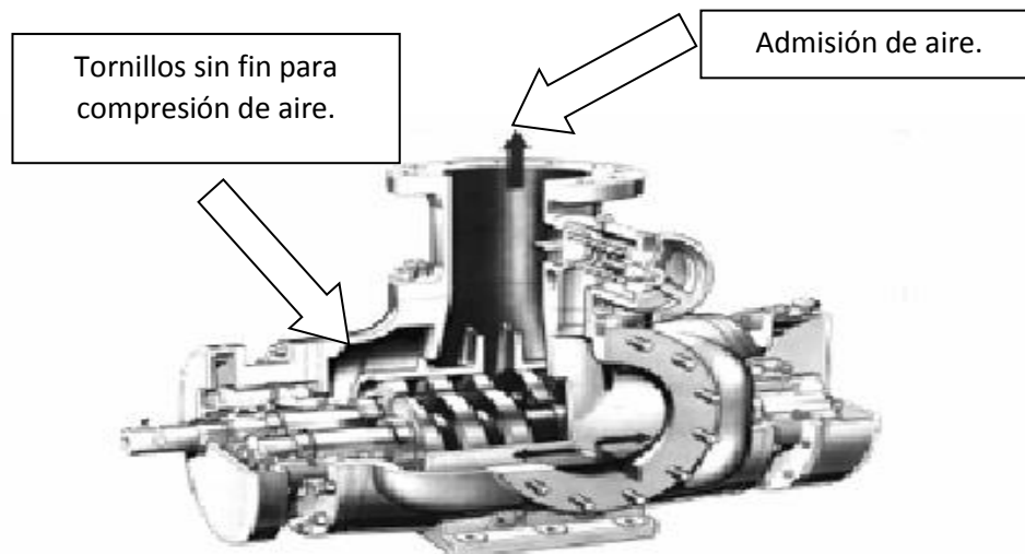
Figura 6. Compresor de Husillo o de Tornillo (CDP)
