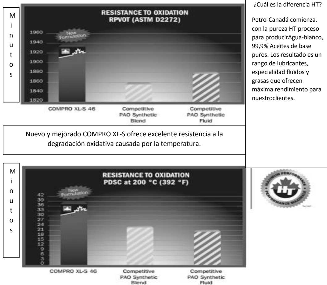
Figura 32. Resistencia del aceite con respecto al tiempo de trabajo
