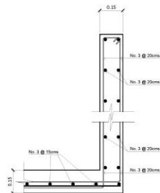
SECCION A-A' PLANTA DE TRATAMIENTO
