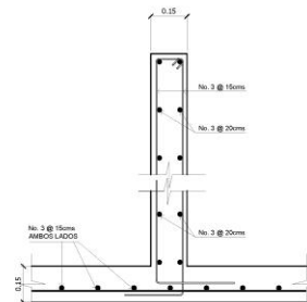
SECCION B-B' PLANTA DE TRATAMIENTO
