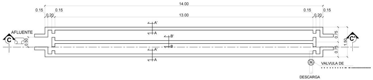
PLANTA DE 2 DESARENADORES PLANTA DE TRATAMIENTO
